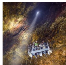
9. Príhnúkagigur
